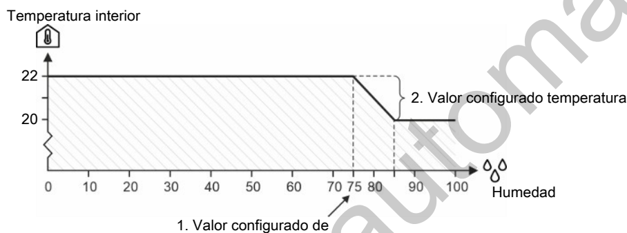
Figura 12: Control de humedad con reducción de temperatura
