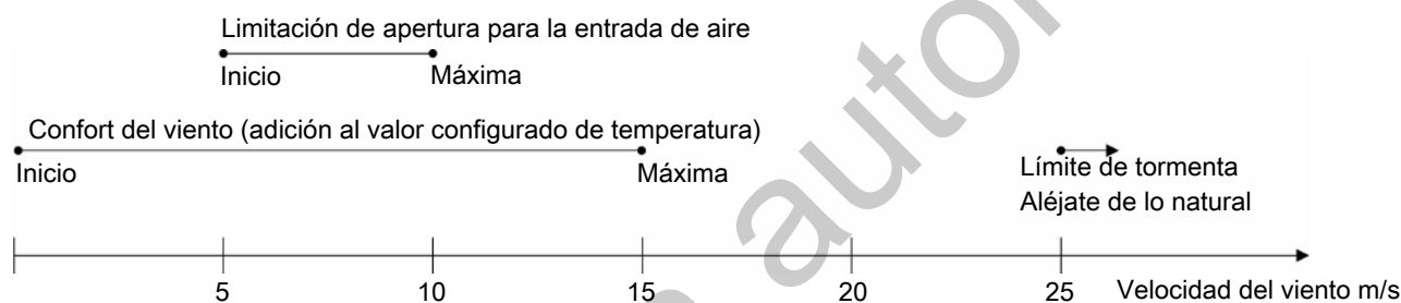
Figura 21: Ventilación natural con velocidad del aire en aumento
