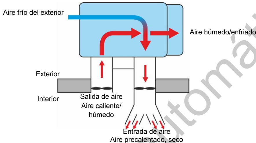
Figura 14: Ejemplo de principio de unidad recuperadora de calor.
