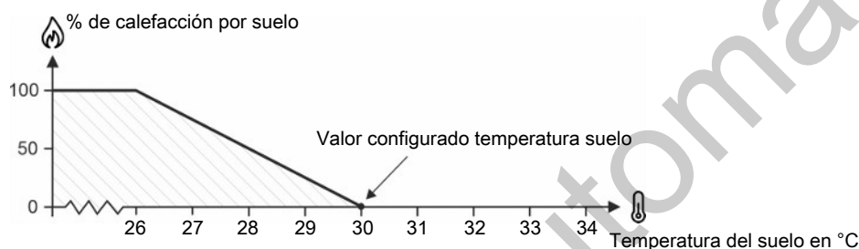
Figura 36: Calefacción por suelo con sensor de temperatura
