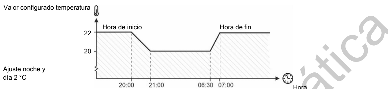
Figura 8: Ajuste de día y noche establecido como un descenso nocturno de la temperatura.
