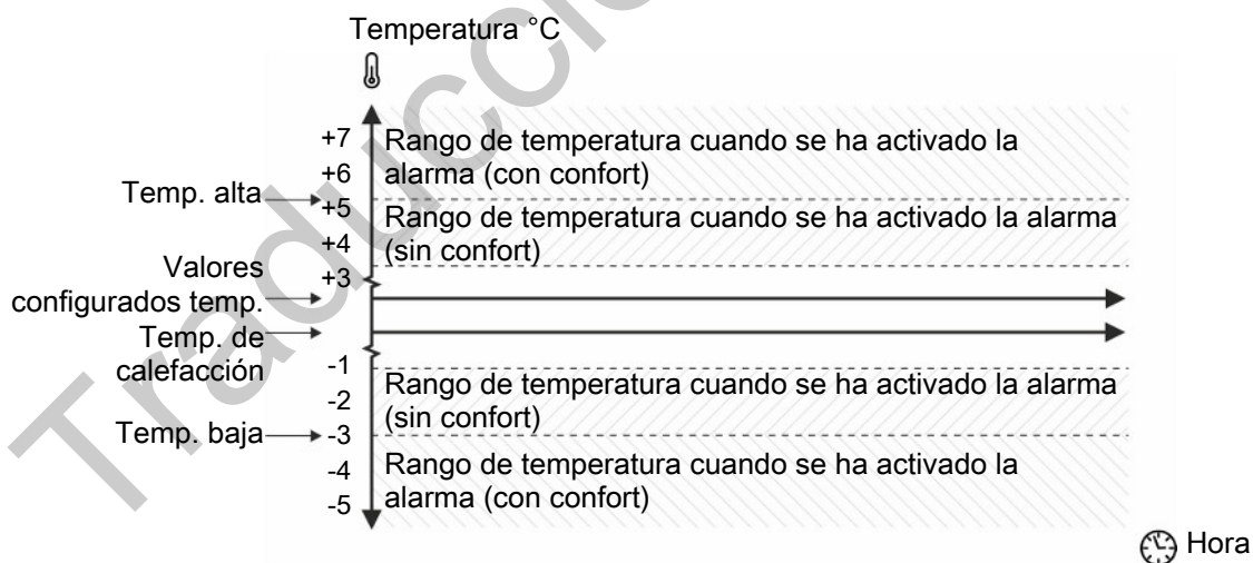
Figura 41: Alarma de temperatura alta y baja
