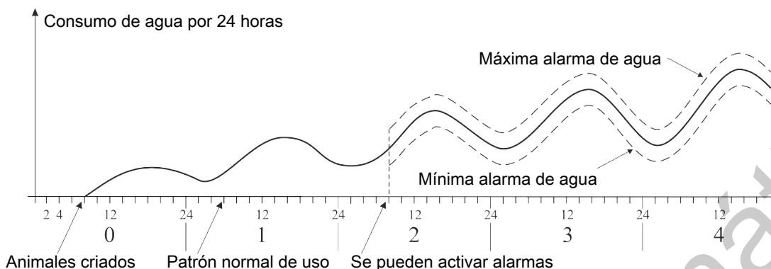
Figura 43: Ejemplo de alarmas de agua mín. y máx.
