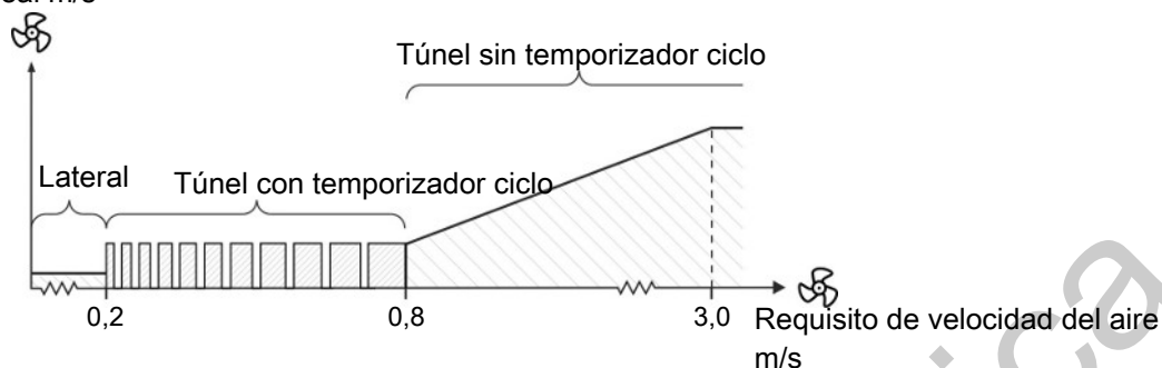
Figura 16: Secuencia de ventilación con temporizador de ciclo en la ventilación de túnel.
