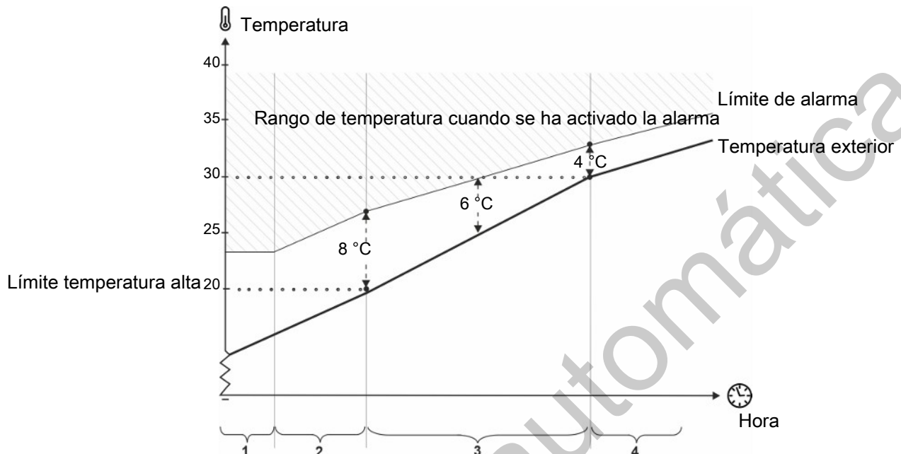
Figura 42: Temperatura de verano a 20 °C y 30 °C en el exterior
