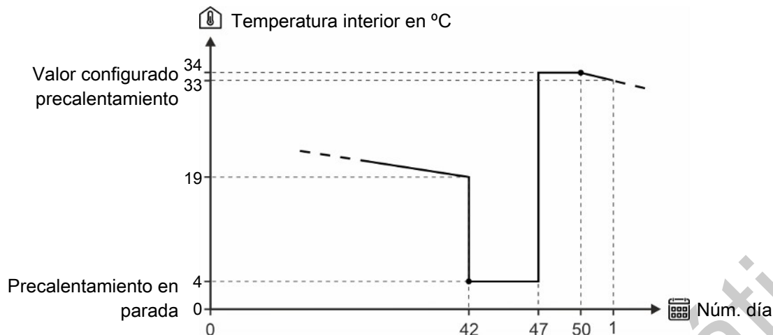
Figura 38: Ejemplo de ajuste de precalentamiento.
