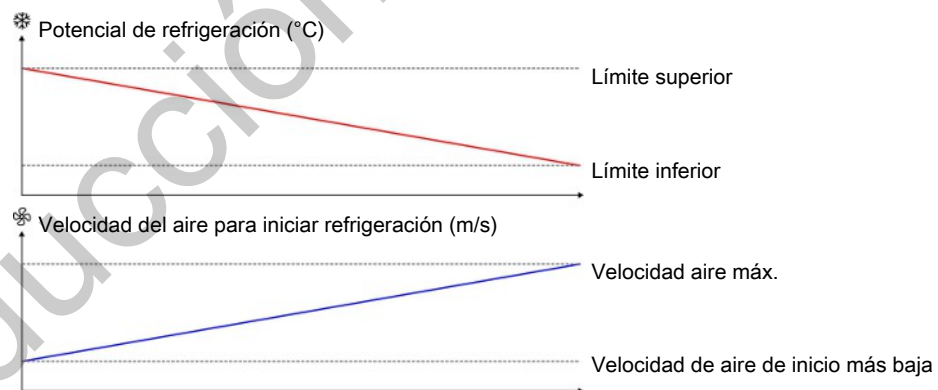
Figura 31: En áreas con baja humedad exterior y un gran potencial de refrigeración, este puede comenzar a una velocidad de aire más baja. Mientras que en áreas con bajo potencial de refrigeración, este comenzará lo más tarde posible, es decir, a la velocidad del aire máxima.
