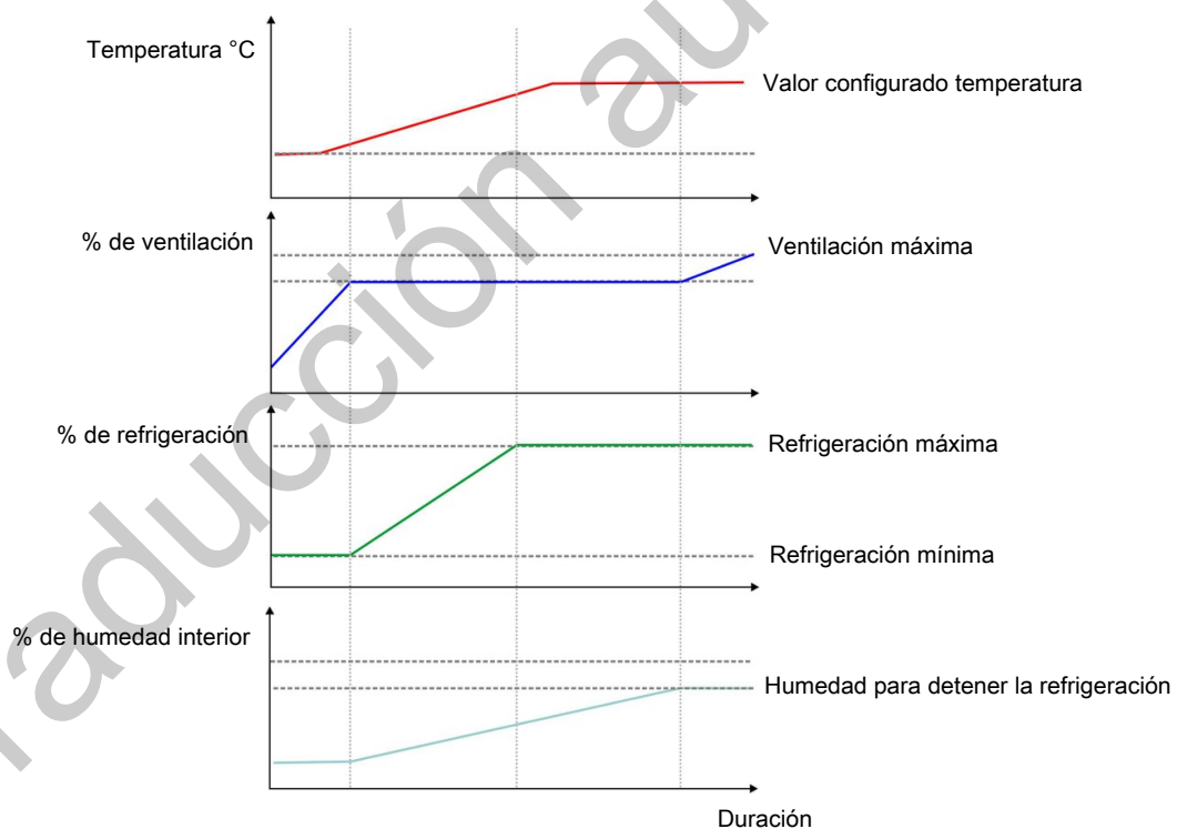
Figura 25: Para mantener la temperatura interior requerida, la refrigeración comenzará antes de que el nivel de ventilación haya alcanzado la ventilación máxima. Cuando la refrigeración no puede mantener la temperatura, la ventilación aumentará nuevamente.
