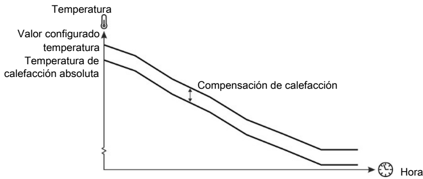
Figura 33: Establecer compensación de calefacción
