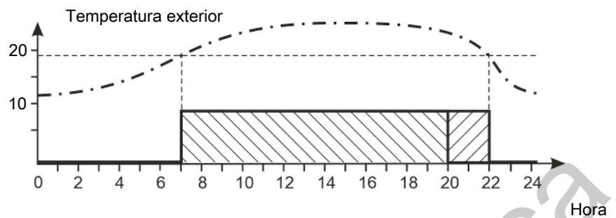
Figura 30: Pulverización según la hora y la temperatura exterior
