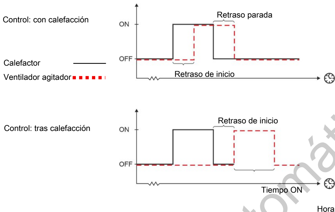
Figura 23: Control con calefacción
