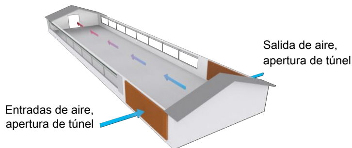
Figura 19: Ejemplo de nave ganadera con ventilación natural en combinación con ventilación túnel, ventilación túnel.
