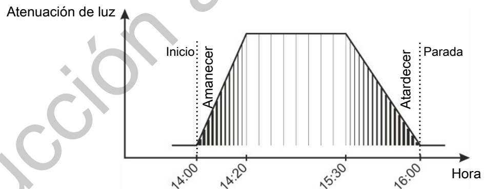
Figura 39: Atenuación de luz normal El amanecer y el atardecer se integran en el periodo de luz.
