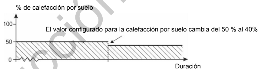
Figura 37: Calefacción por suelo sin sensor de temperatura
