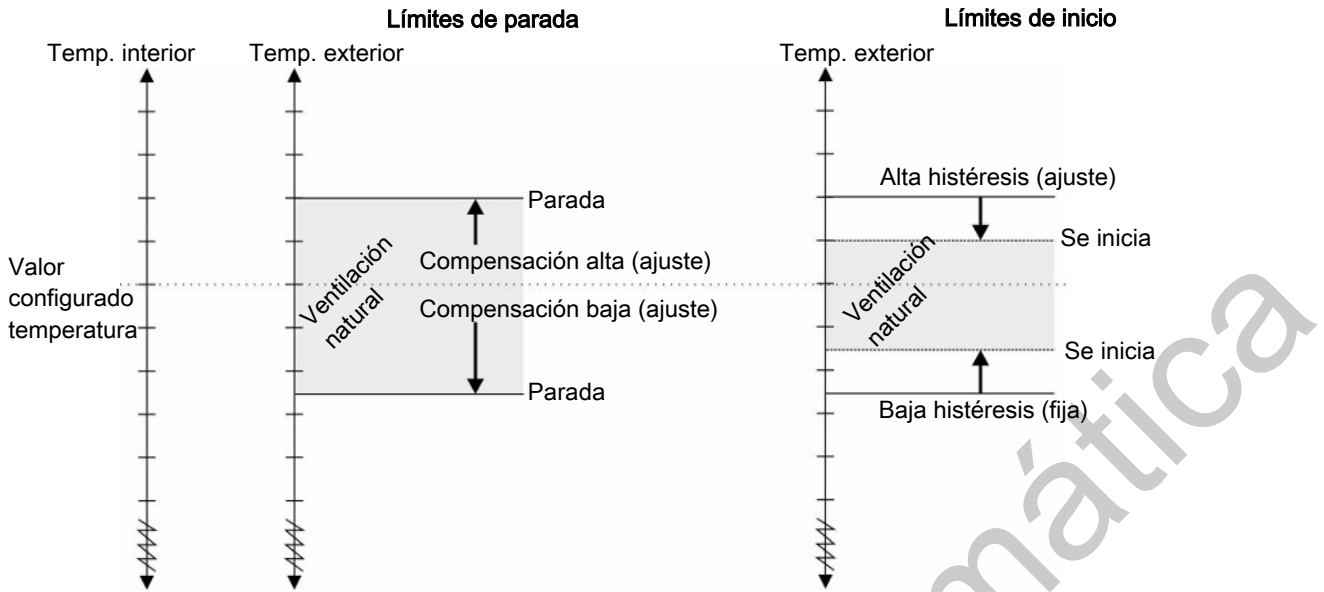
Figura 20: Iniciar y detener en relación con la temperatura exterior. Los límites de temperatura se establecen como compensados con el valor configurado de temperatura.
