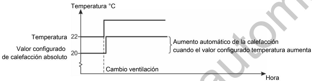
Figura 34: Suministro de calor
