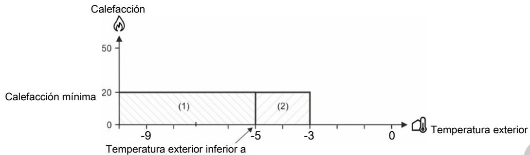
Figura 35: Calefacción mínima al reducirse o incrementarse la temperatura exterior
