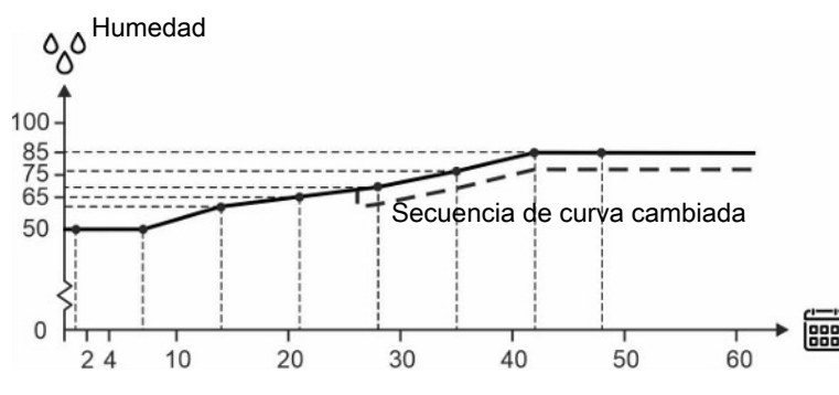
Figura 3: Curva para la humedad del aire
